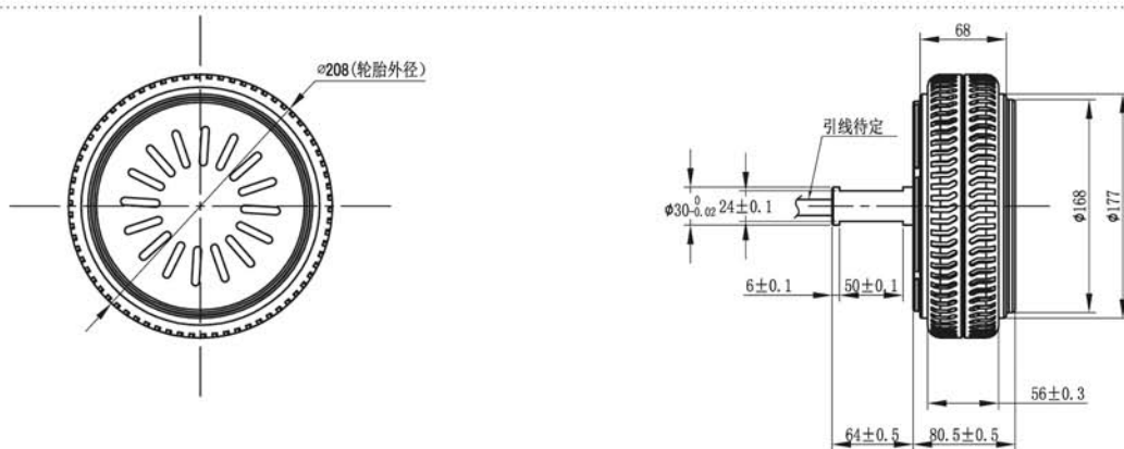
直流无刷电机 BLDC MOTOR
